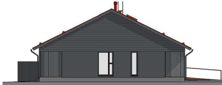
PÄÄTY ITÄÄN
