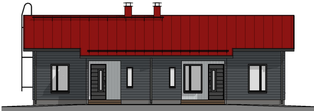
JULKISIVU POHJOISEEN
